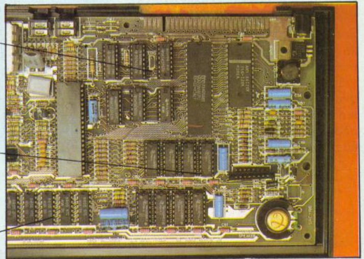
Chips ampliación memoria TMS 4532 (L3/ L4)
